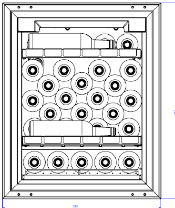
V-INSP-S Pack access 30 bouteilles/bottles
